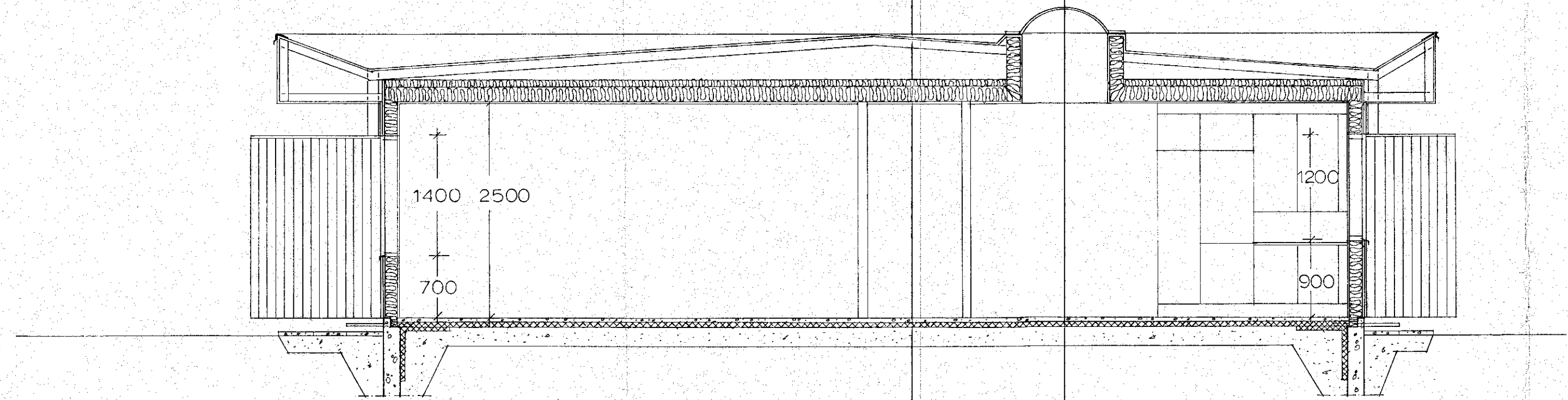
leikkaus A - A
