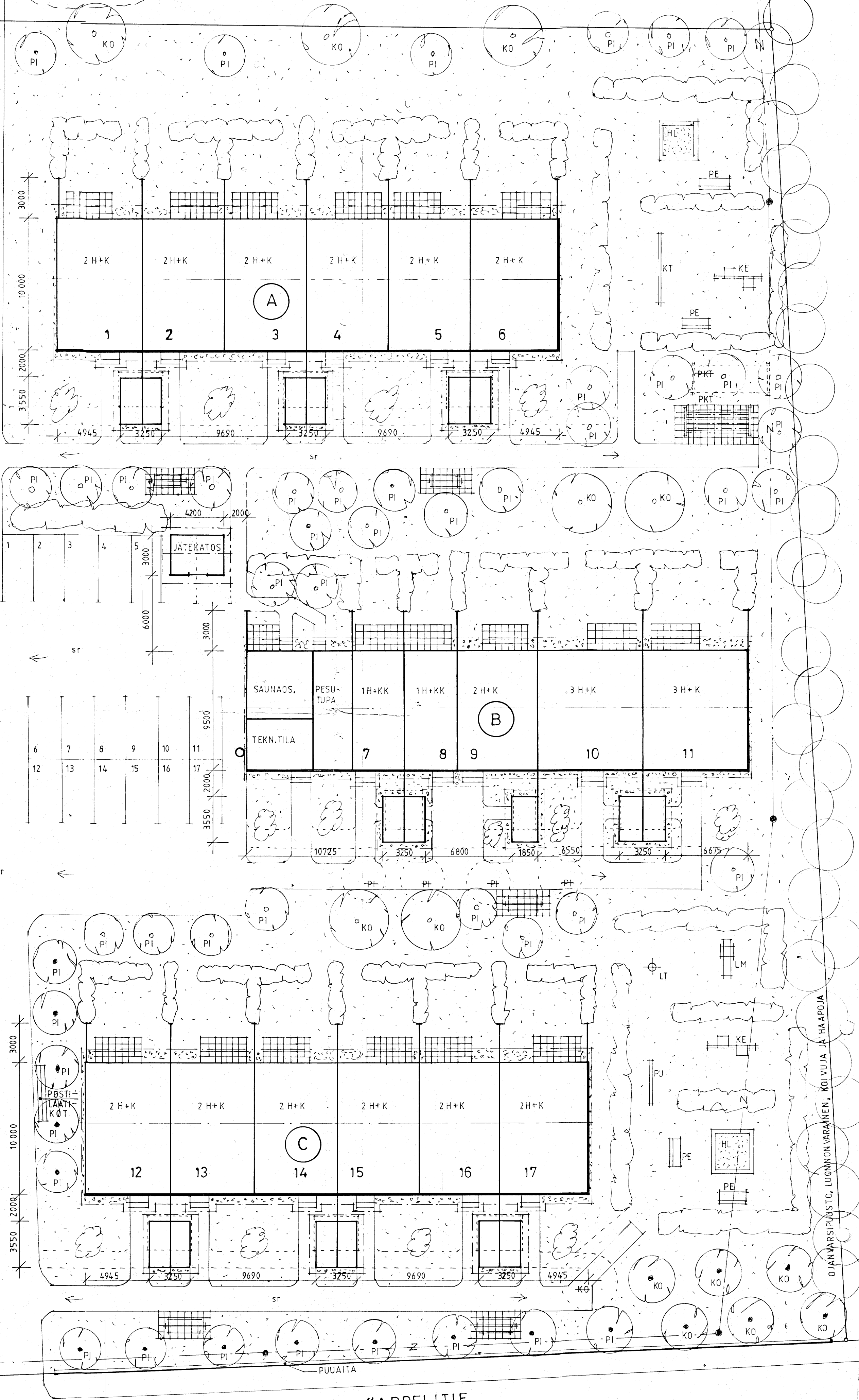
ASEMAPIIROS 1:200
